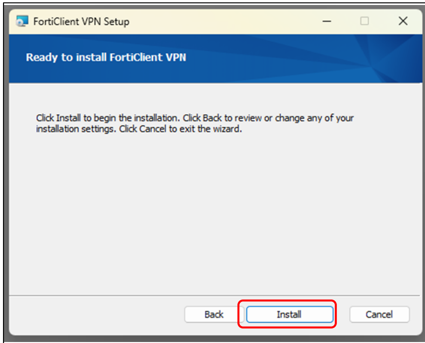
図 6-1-10 Setup 画面 2
