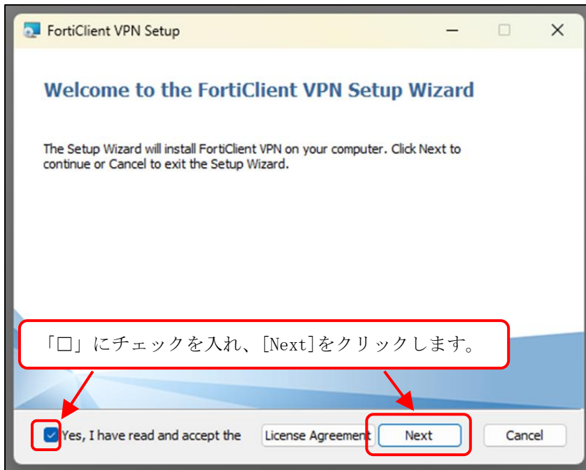
図 6-1-23 Setup 画面 1
