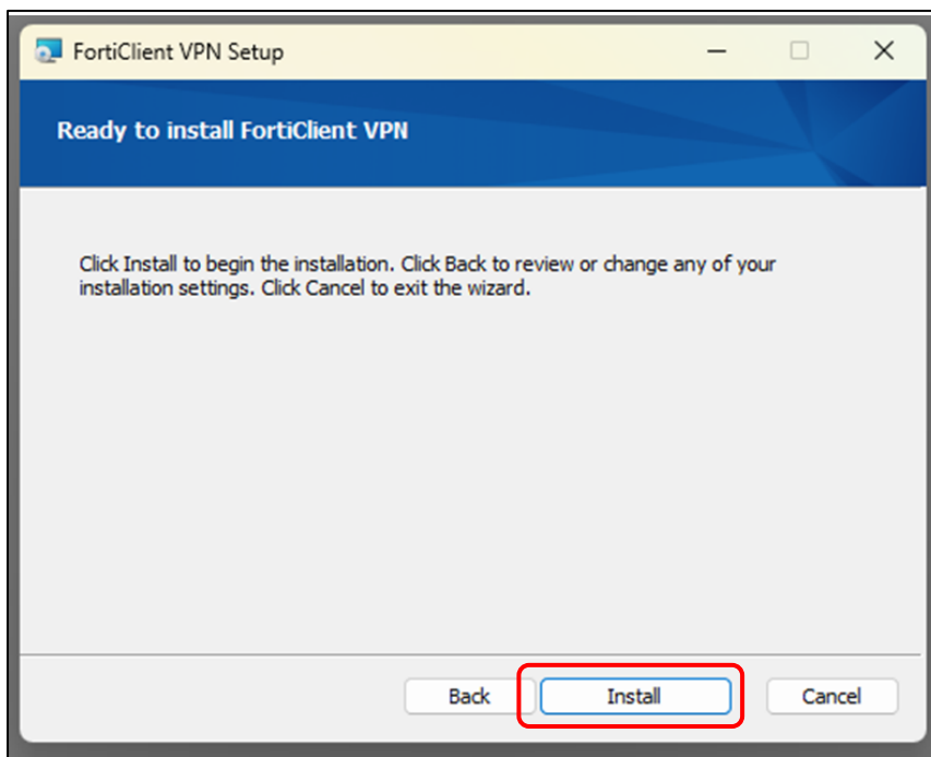
図 6-1-24 Setup 画面 2
