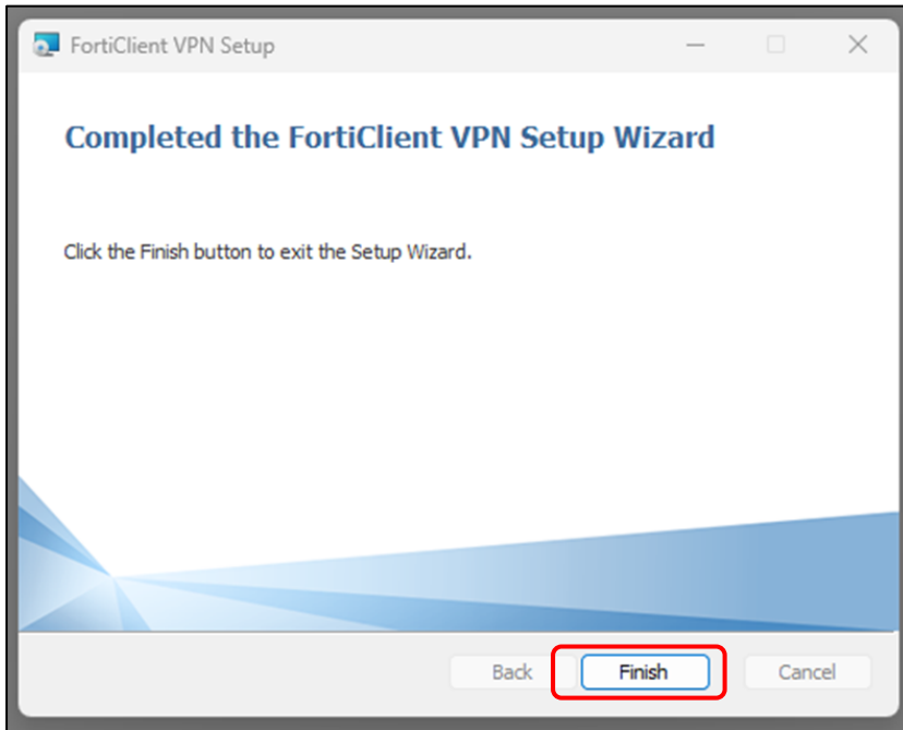
図 6-1-25 Setup 画面 3
