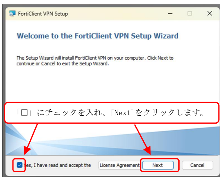
図 6-1-9 Setup 画面 1
