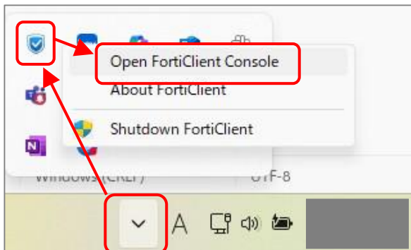
図 6-1-12 FortiClient を起動
