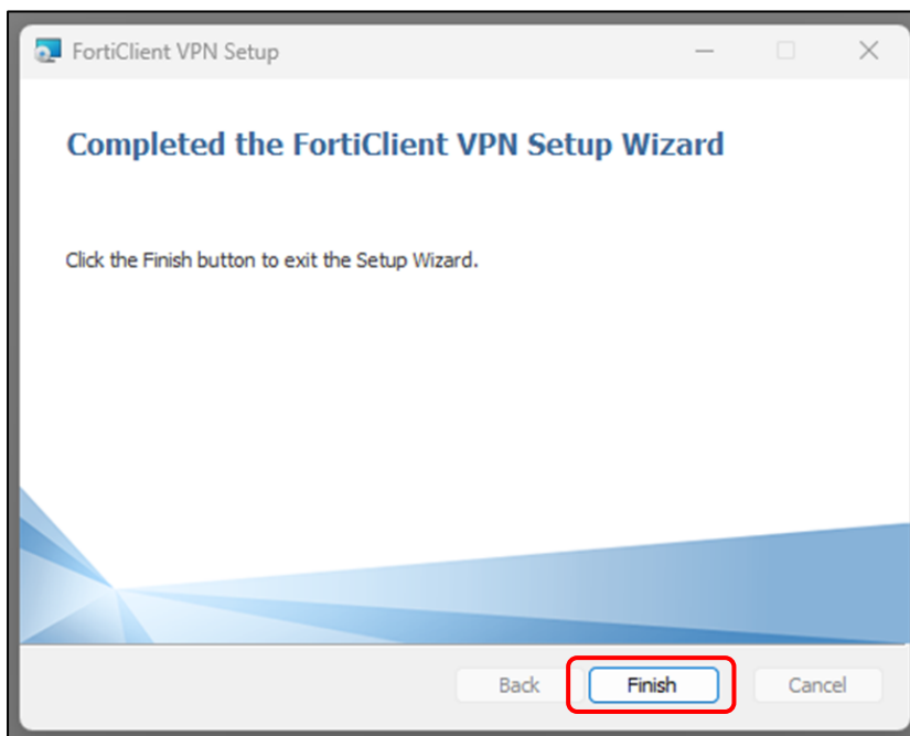
図 6-1-11 Setup 画面 3
