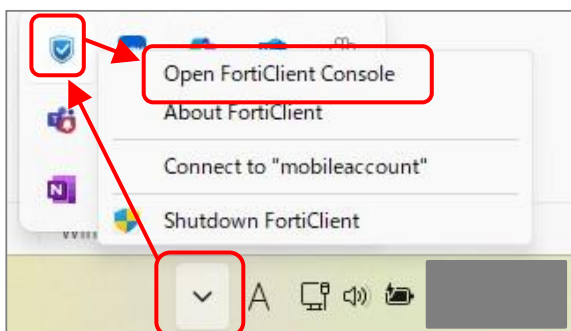
図 7-1-12 FortiClient を起動
