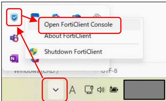
図 6-1-26 FortiClient を起動
