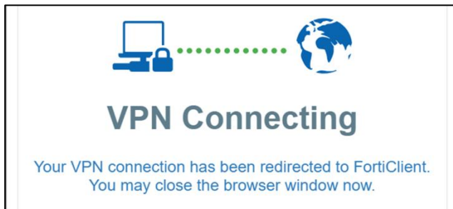
図 7-1-7 SSL-VPN 接続中
