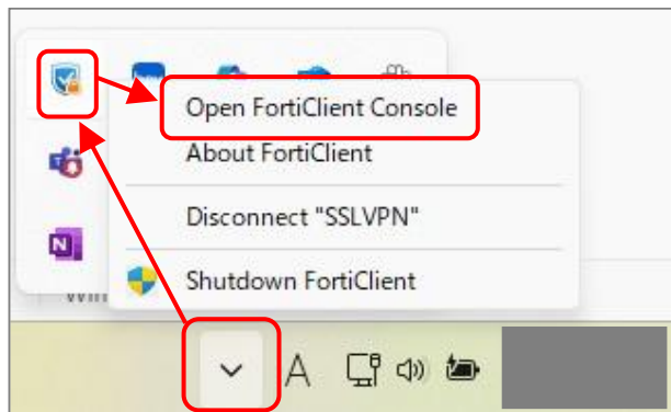
図 7-2-1 FortiClient を起動
